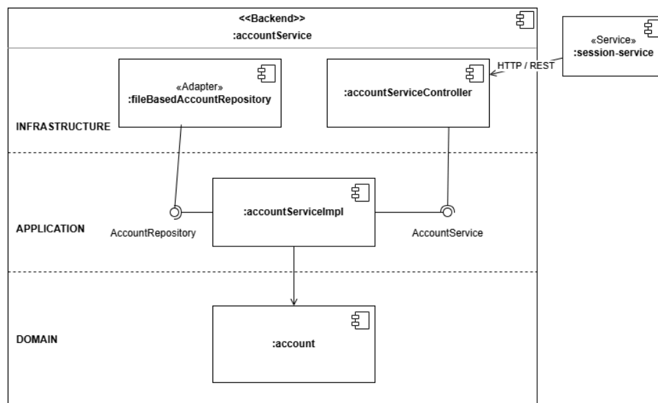
C&C diagram dell'account service
